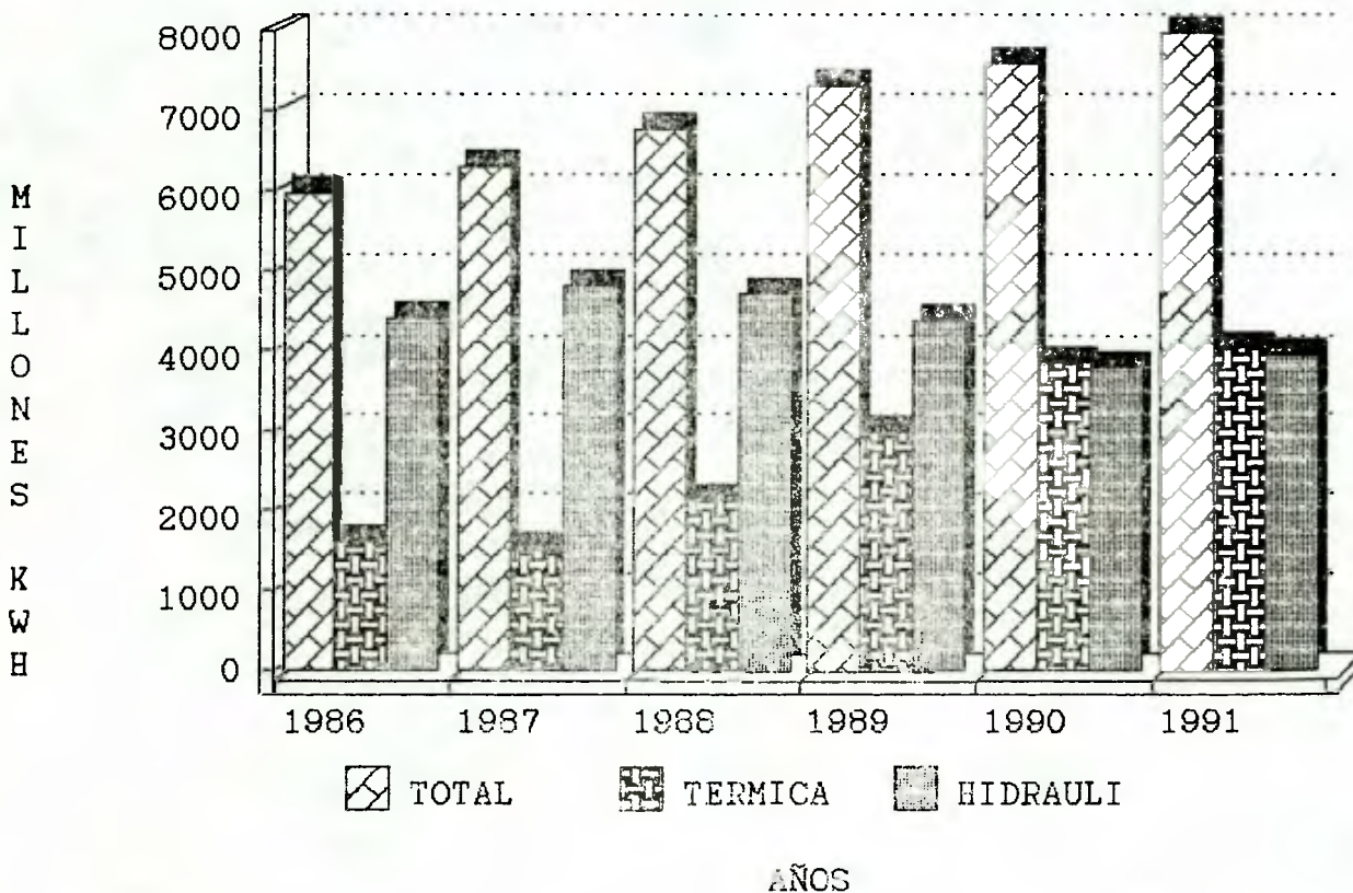
GENERACION DE ENERGIA ELECTRICA ENERO - MAYO 1986 - 91
