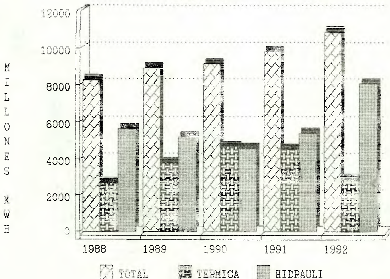
GENERACION DE ENERGIA ELECTRICA ENERO - JUNIO 1988 - 92
